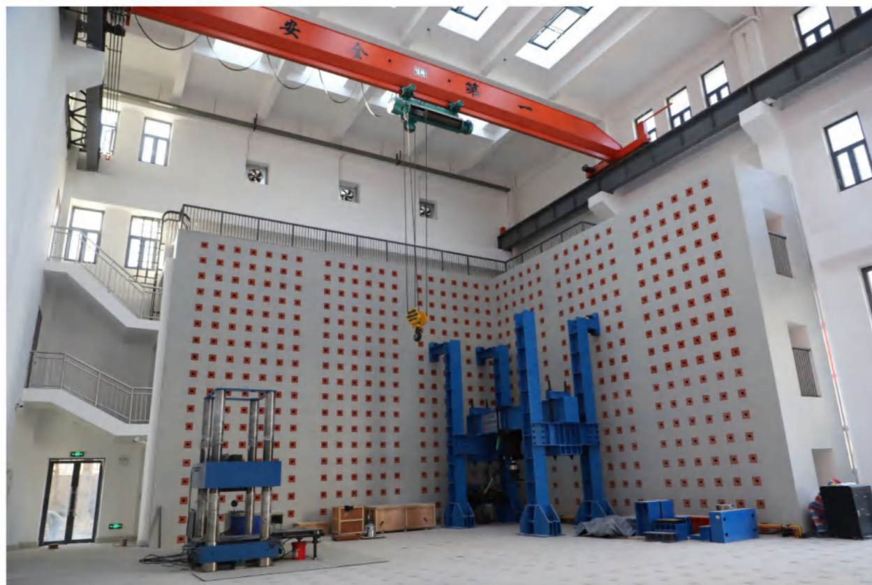
多通道电液伺服加载系统 ▼
